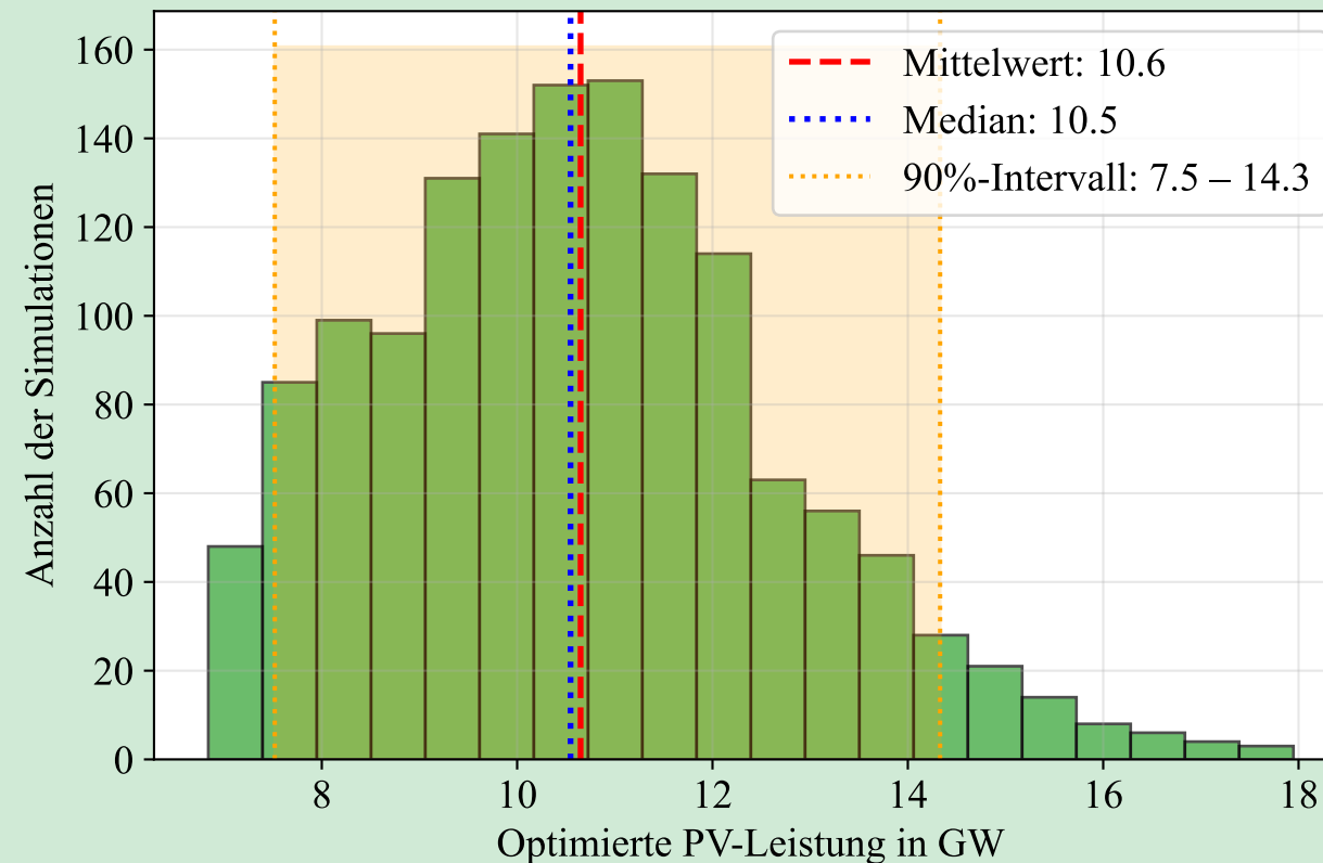
3. Unsicherheit Optimierte PV-Leistung aus 1,400 Simulationen
