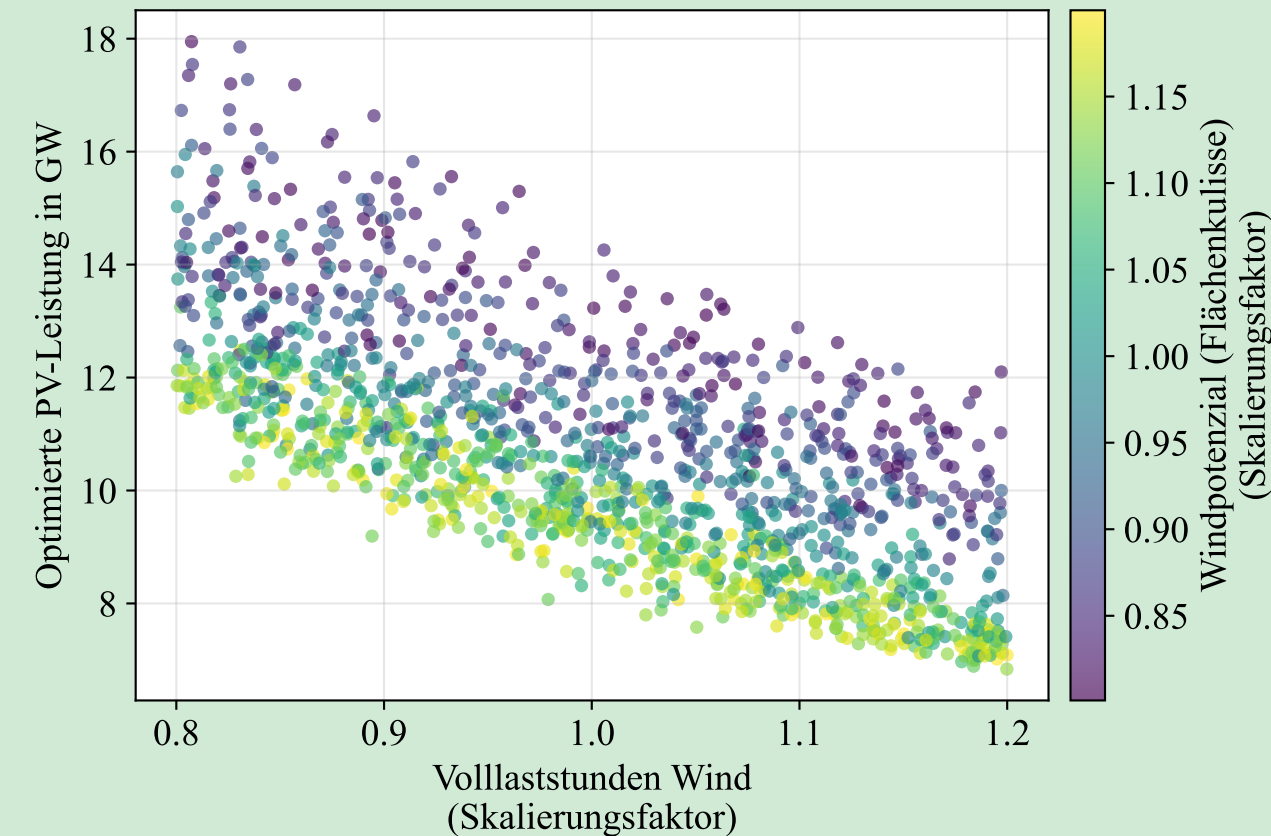
4. Parameterinteraktion Volllaststunden Wind vs. Windpotenzial (Flächenkulisse)
